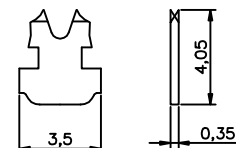
平面二叉标准端子
