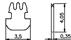
平面三爪端子
