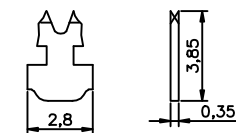
平面二叉小端子
