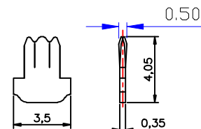
三叉端子
